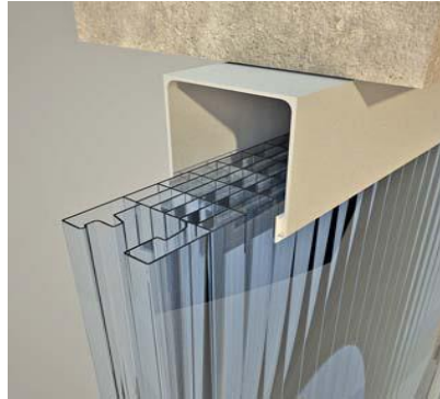
oberes Rahmenprofil
